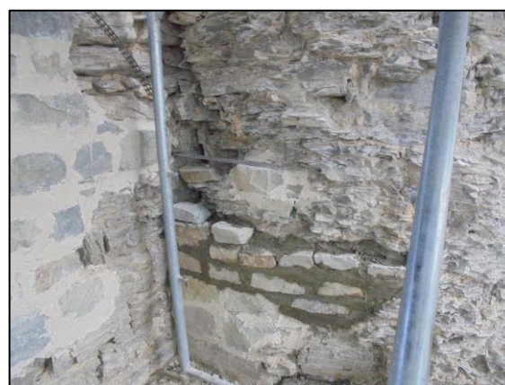
Verlegen der Edelstahl-Bandbewehrung (oben), und Mauerwerkergänzung am Turmschaft (unten).
